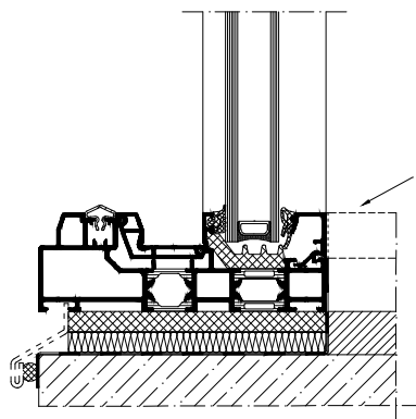
Anslutningsprincip i lyftskjutsystem
