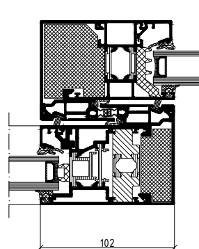
Mittmöte i lyftskjutsystem
