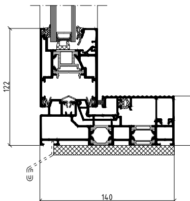
Profilmått i lyftskjutparti
