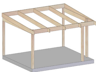
VPP Pulpet 4, brutet hörn (x1)
