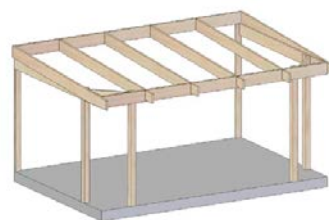
VPP Pulpet 5, brutet hörn (x2)
